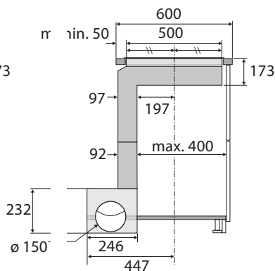
Zijaanzicht gedraaide motor
