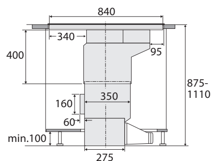
Voorraanzicht
