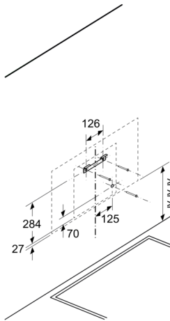
Afmeting in mm Wandinstallatie zonder luchtkanaal:
