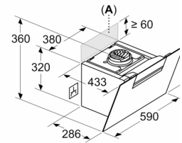
Afmeting in mm Apparaat in luchtcirculatiemodus kanaal
