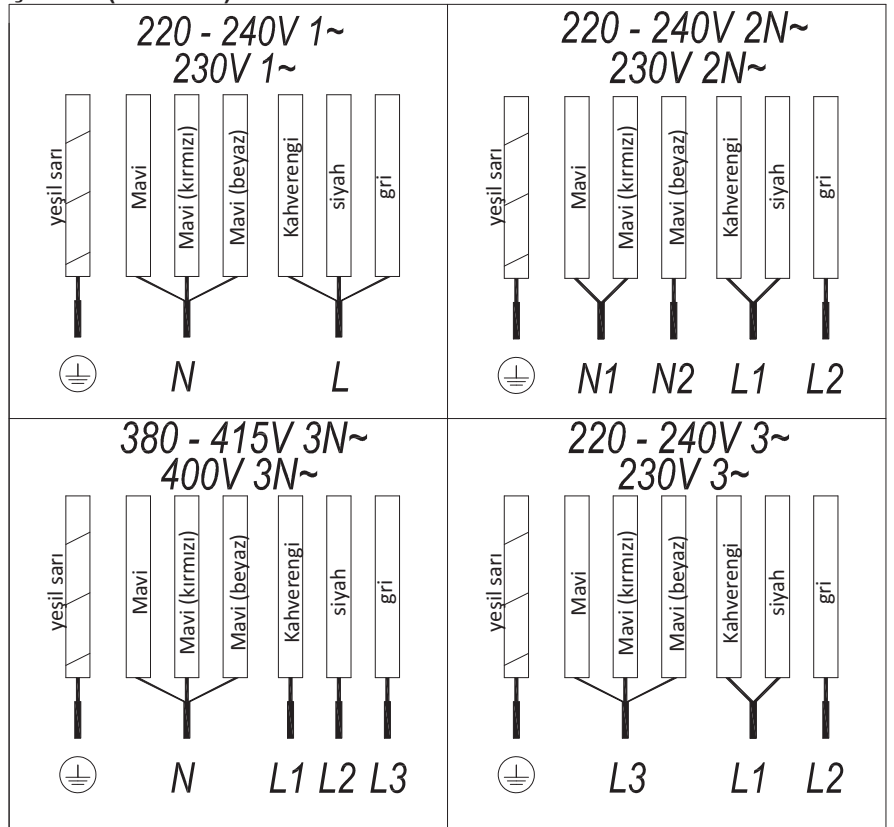
Şekil 2b (7 KABLO)
