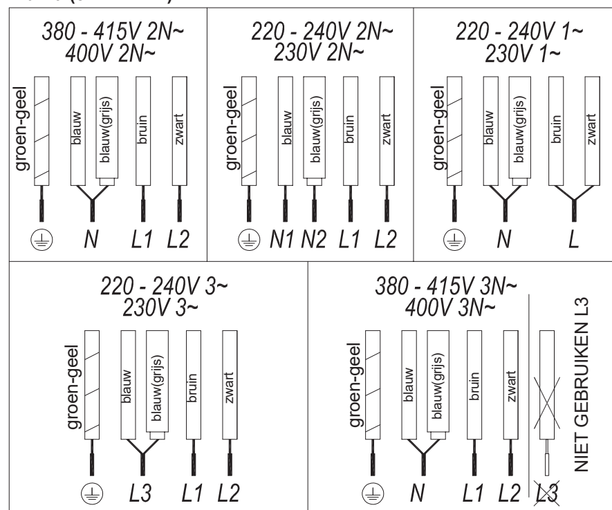
Afb. 2a (5 DRADEN)
